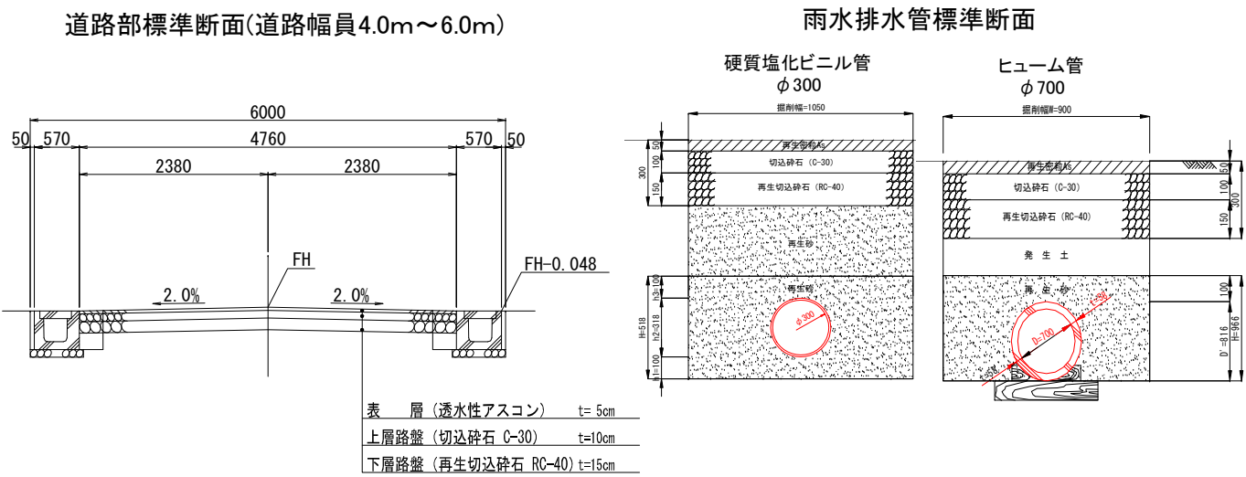
ひょうじゅんだんめんず 標準断面図
